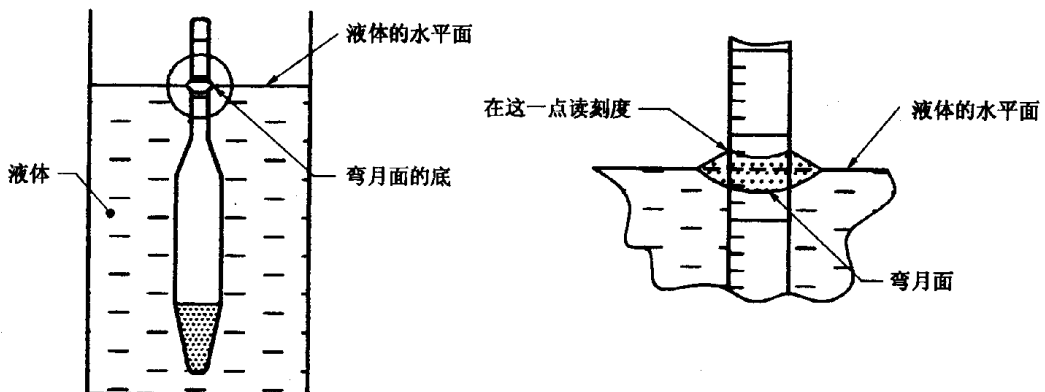
图 1 透明液体的密度计刻度读数
