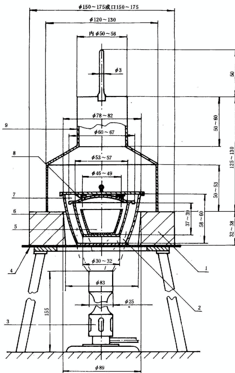
图 1 康氏残炭测定仪
