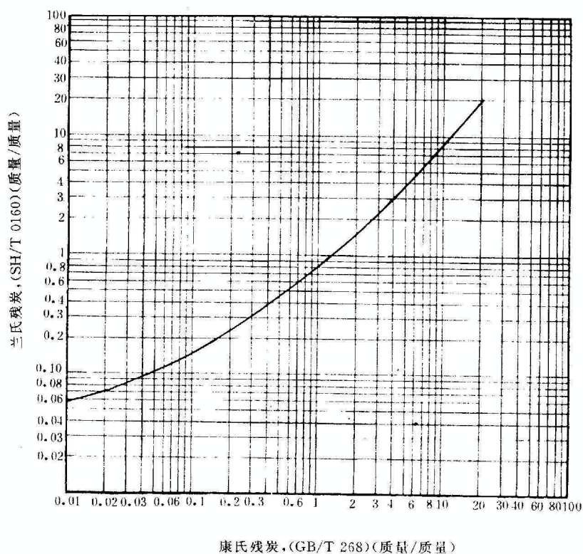
康氏和兰氏残炭值的相互关系图
